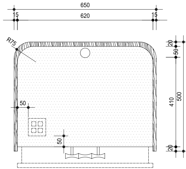
NIGHT STAND PLAN ( RIGHT )
