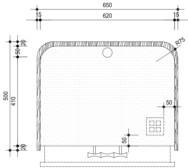
NIGHT STAND PLAN ( LEFT )
