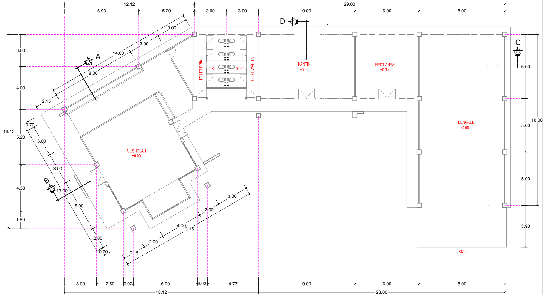
DENAH BANGUNAN PENDUKUNG
