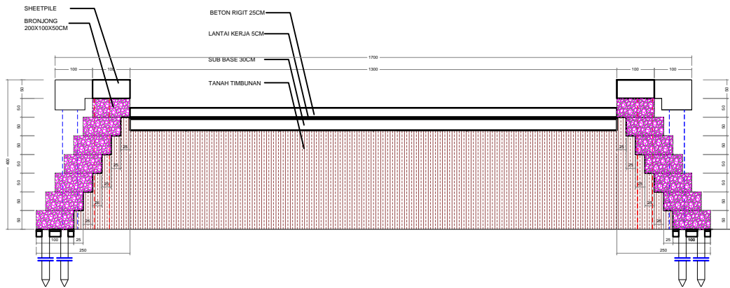
POTONGAN A BERONJONG 1 : 100
