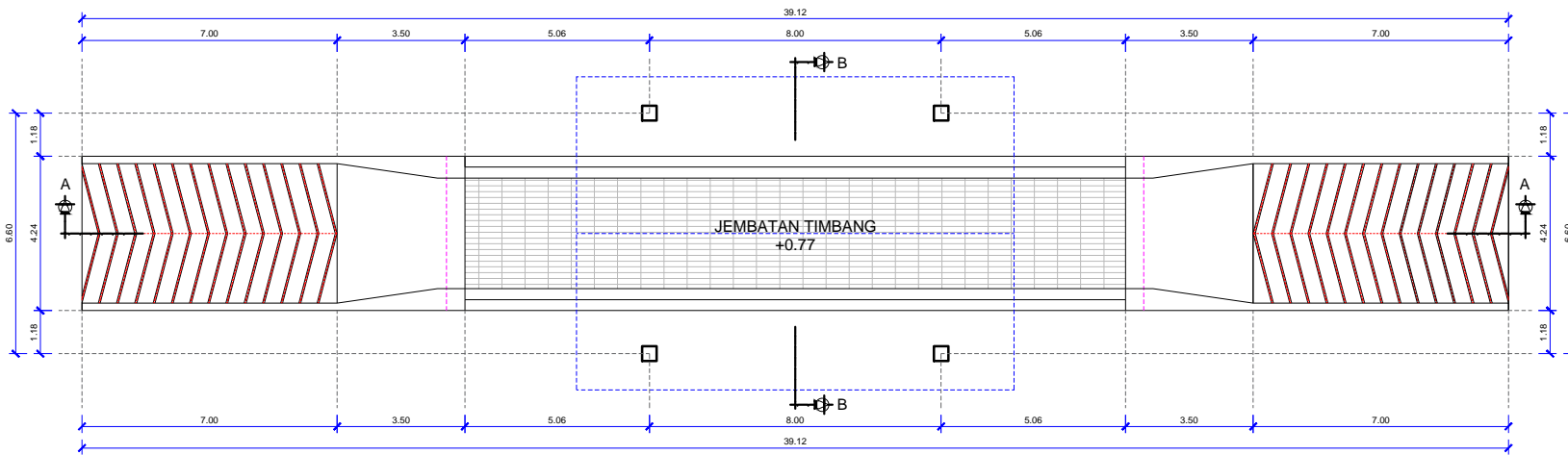
DENAH JEMBATAN TIMBANG skala 1 : 100
