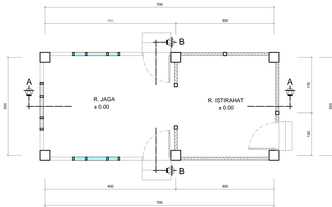
DENAH POS JAGA skala 1 : 50
