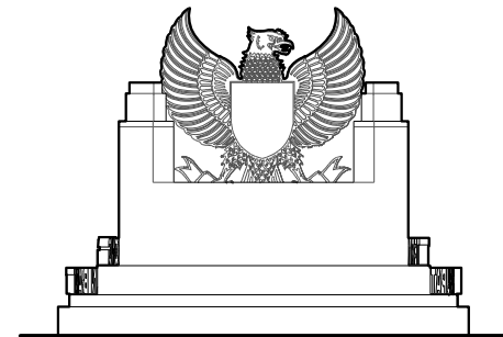
TAMPAK BELAKANG TUGU GARUDA SKALA 1 : 50
