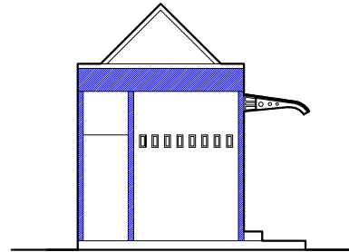
TAMPAK SAMPING KANAN T.WUDHU skala 1:100
