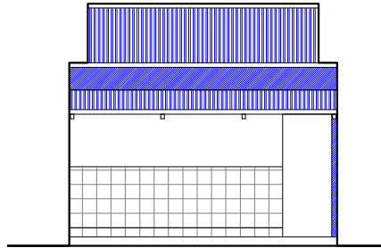
TAMPAK DEPAN T.WUDHU skala 1:100
