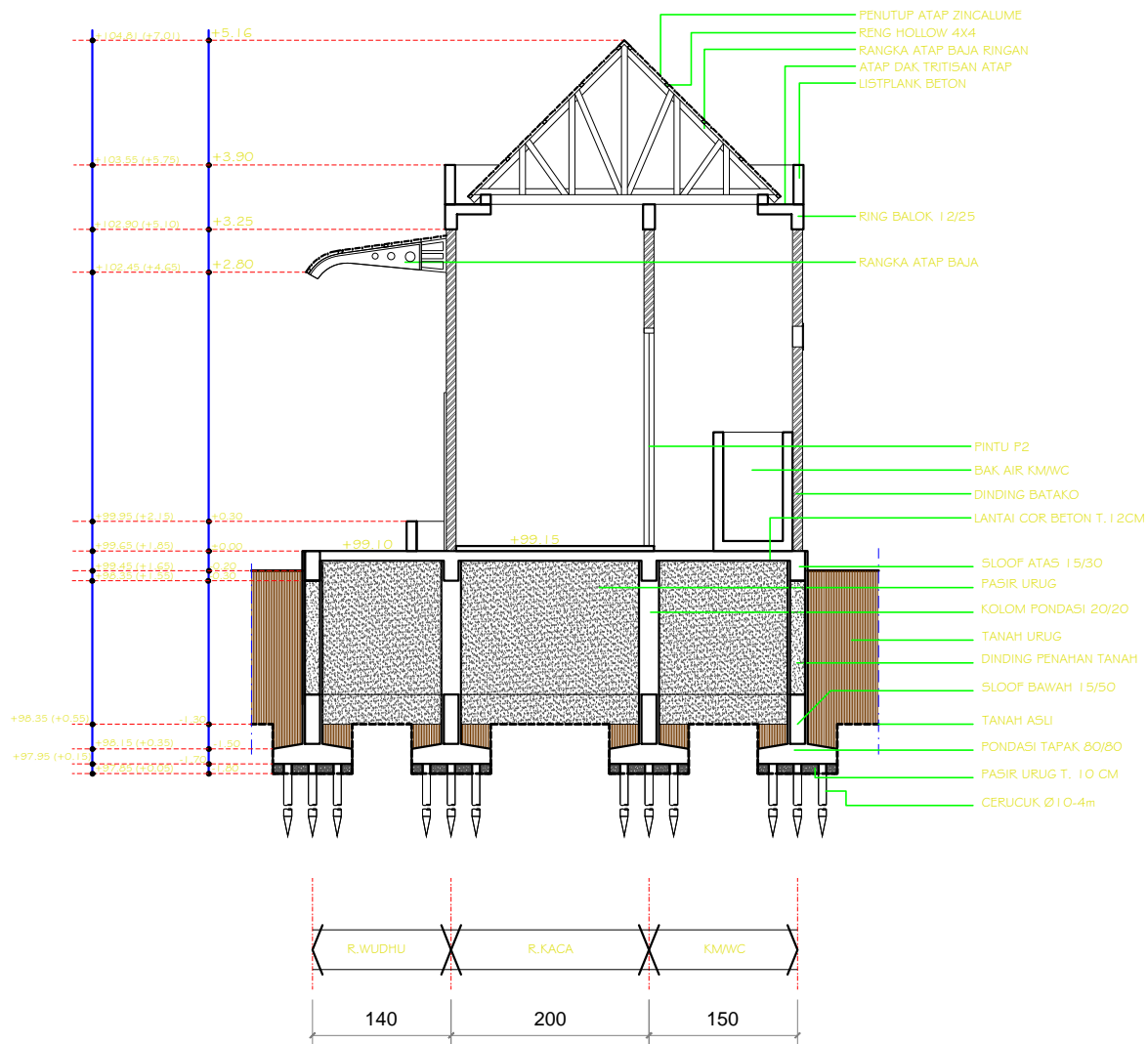
POTONGAN-A T.WUDHU SKALA 1:50
