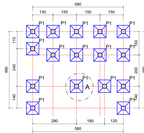
DENAH RENCANA PONDASI T.WUDHU skala 1:100
