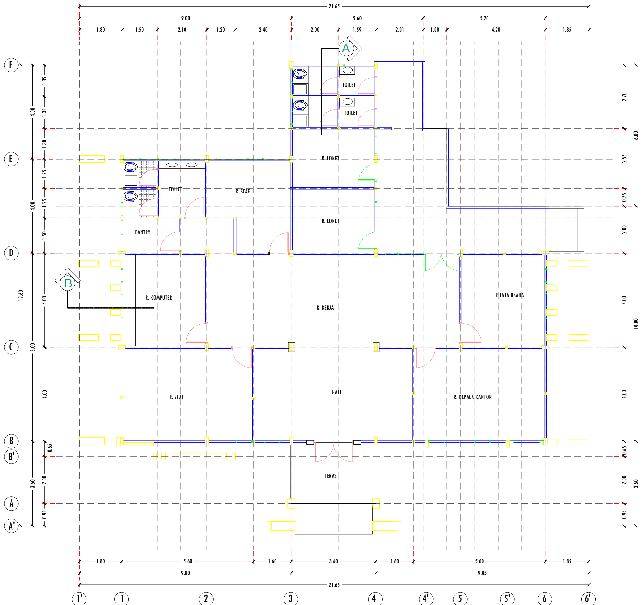
DENAH KANTOR PENGELOLA SKALA 1 : 100
