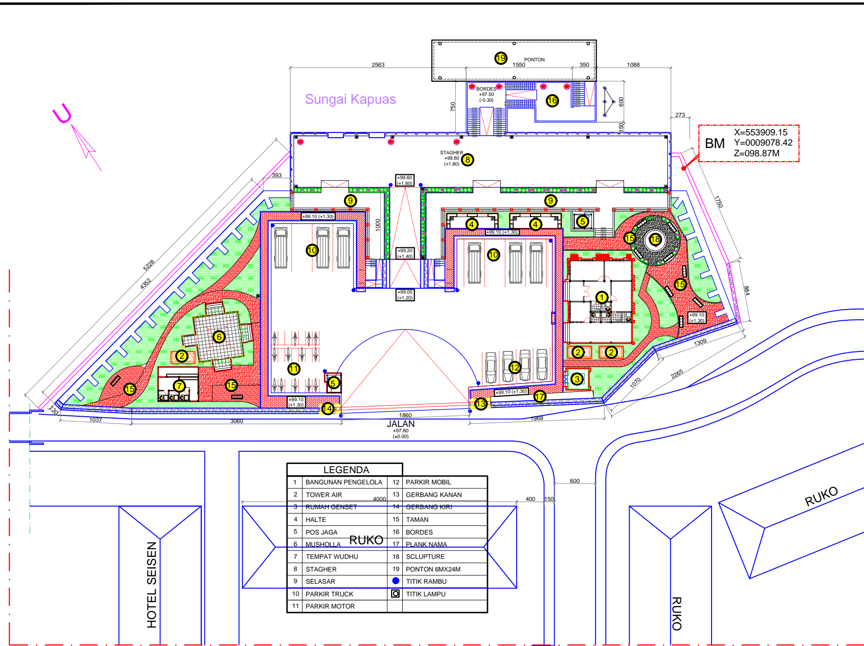
LAYOUT PLAN KETERANGAN DERMAGA SUNGAI DURIAN SKALA 1 : 500
