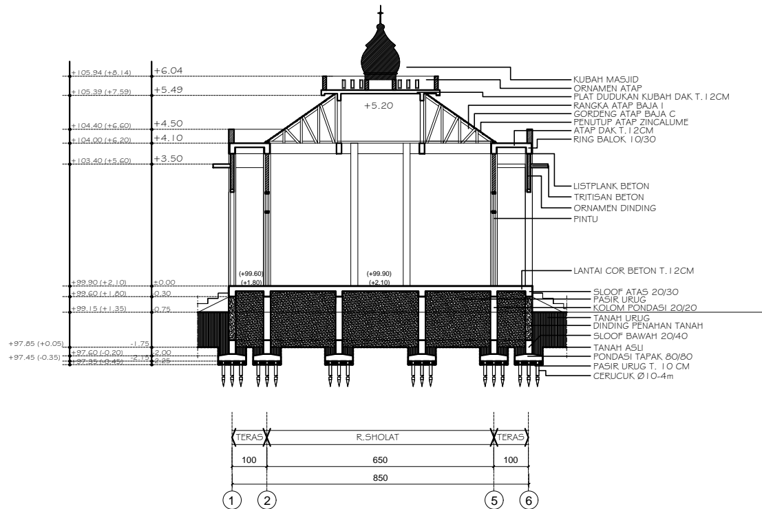
POTONGAN-A MUSHOLLA skala 1:100
