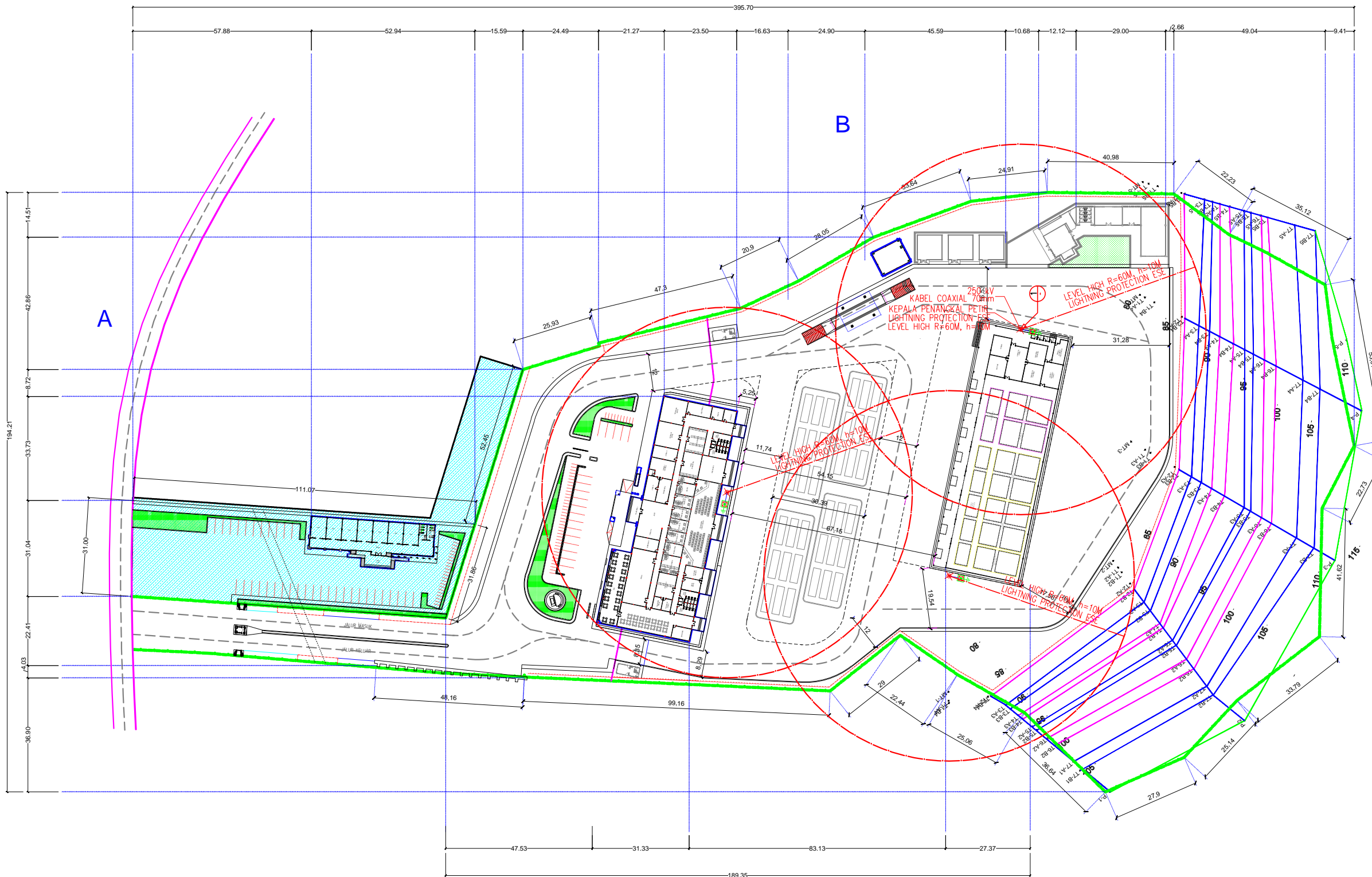
LAYOUT INSTALASI PENANGKAL PETIR SKALA 1 : 1400
