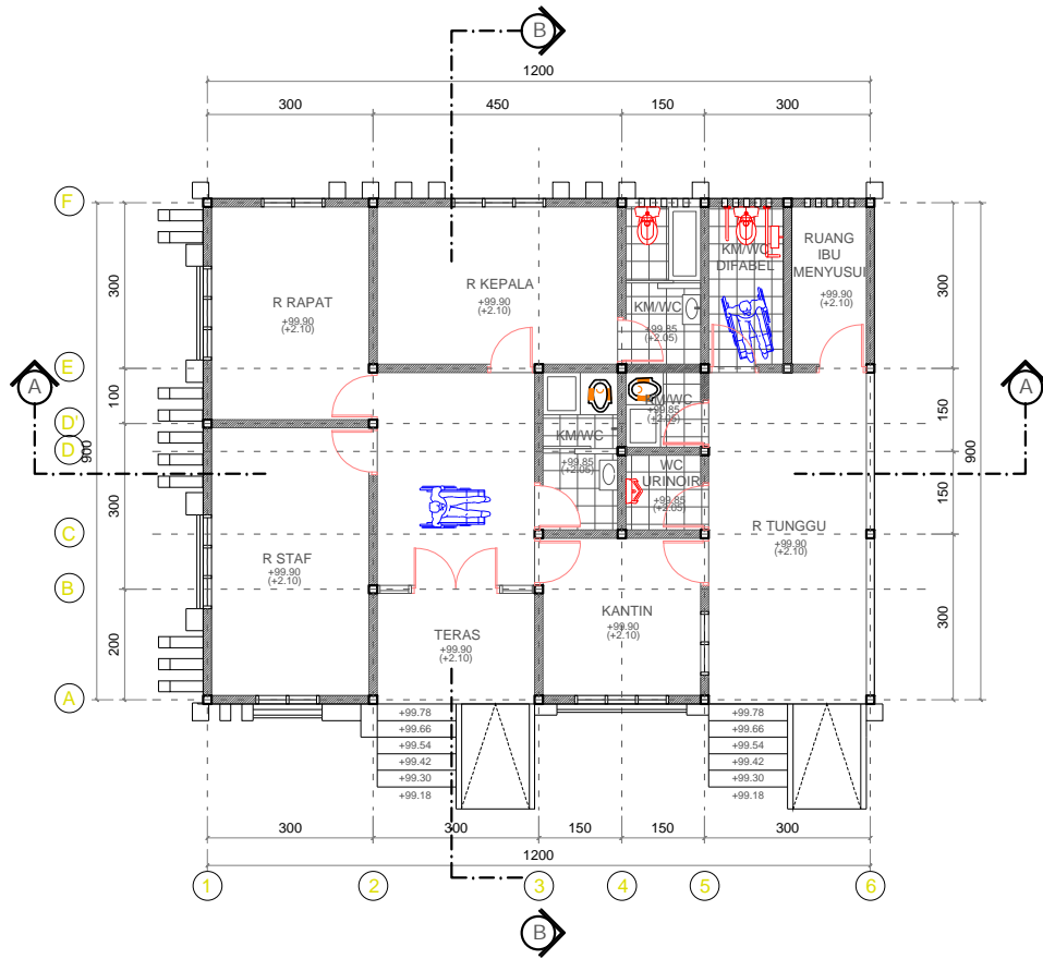
DENAH BANGUNAN PENGELOLA skala 1:100
