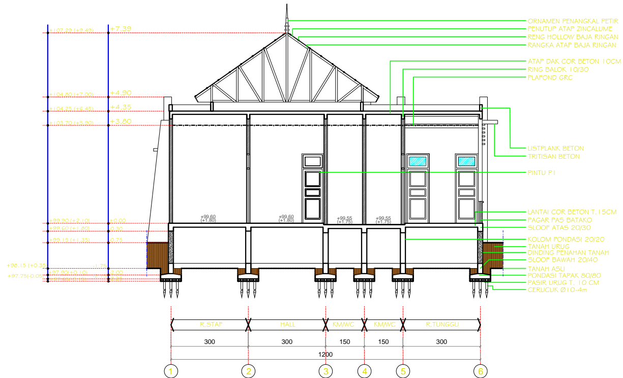
POTONGAN-A BANGUNAN PENGELOLA skala 1:100
