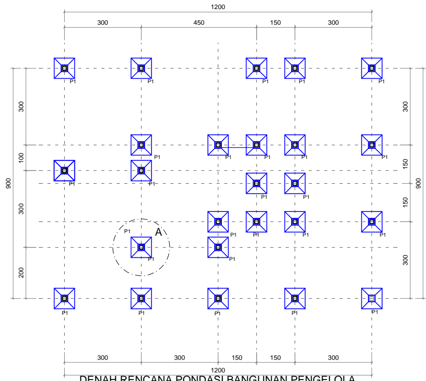
DENAH RENCANA PONDASI BANGUNAN PENGELOLA skala 1:100
