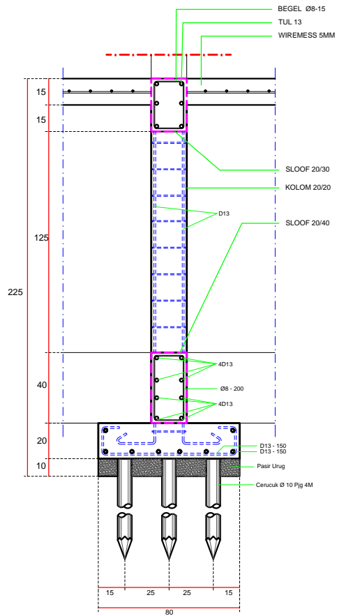
POTONGAN -1 SKALA 1:20
