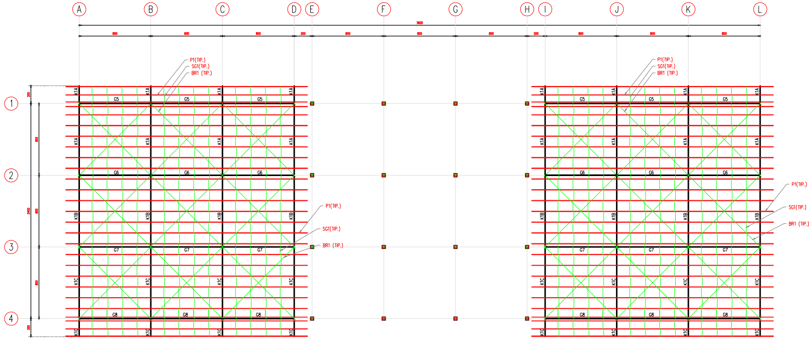
DENAH ATAP (EL+9.200) SKALA 1 : 300
