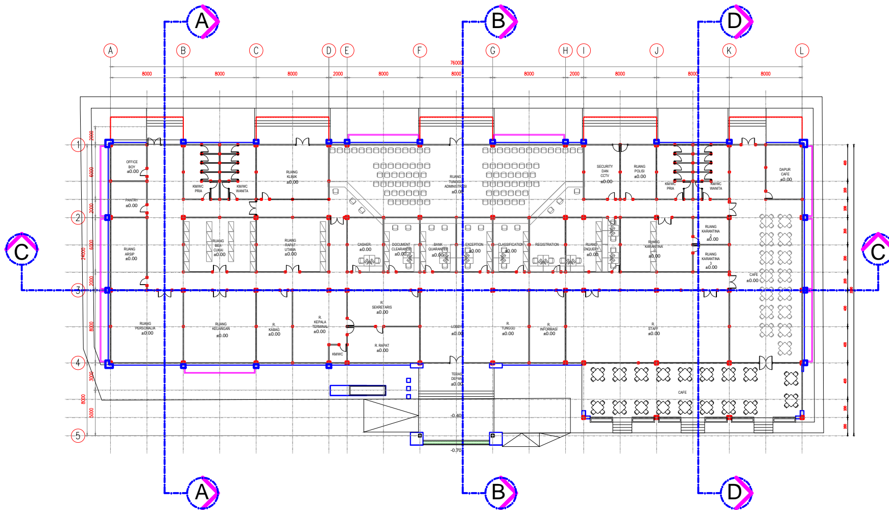
DENAH BANGUNAN KANTOR PENGELOLA SKALA 1 : 300
