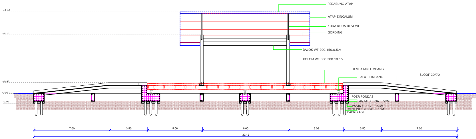
POTONGAN A-A skala 1 : 150
