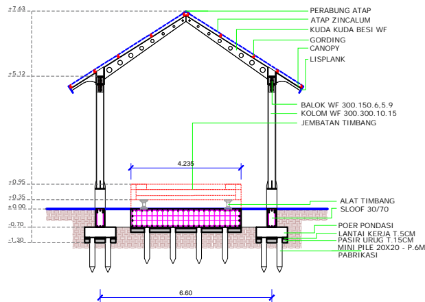
POTONGAN B-B skala 1 : 150
