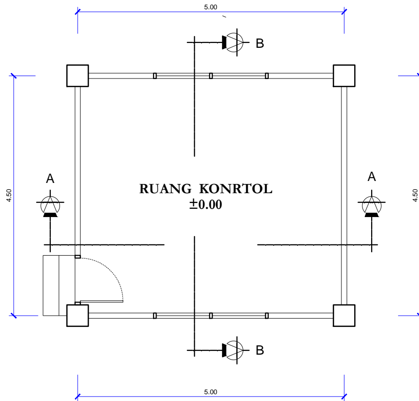
DENAH RUANG KONTROL skala 1 : 50
