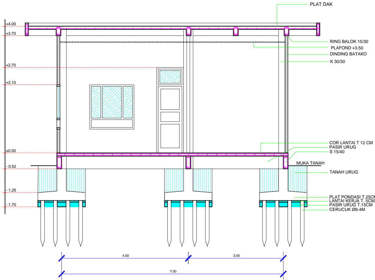
POTONGAN A-A skala 1 : 150
