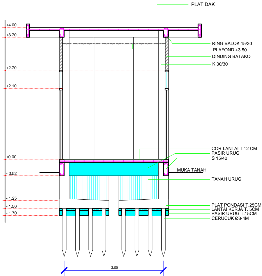
POTONGAN B-B skala 1 : 150
