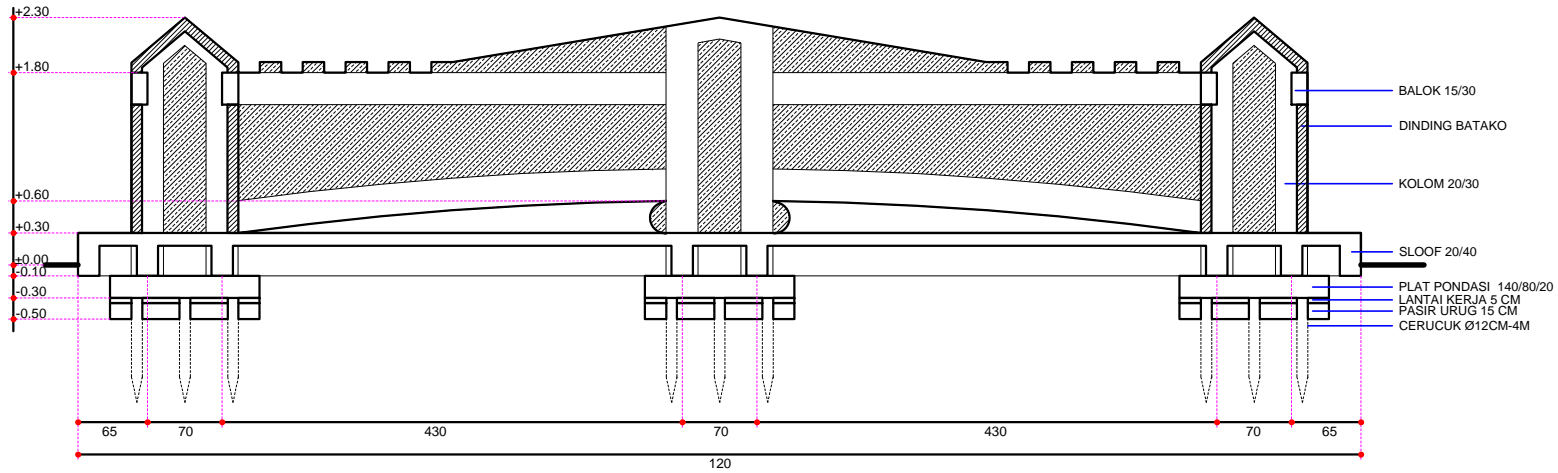
POTONGAN MEMANJANG PLANK NAMA SKALA 1:50
