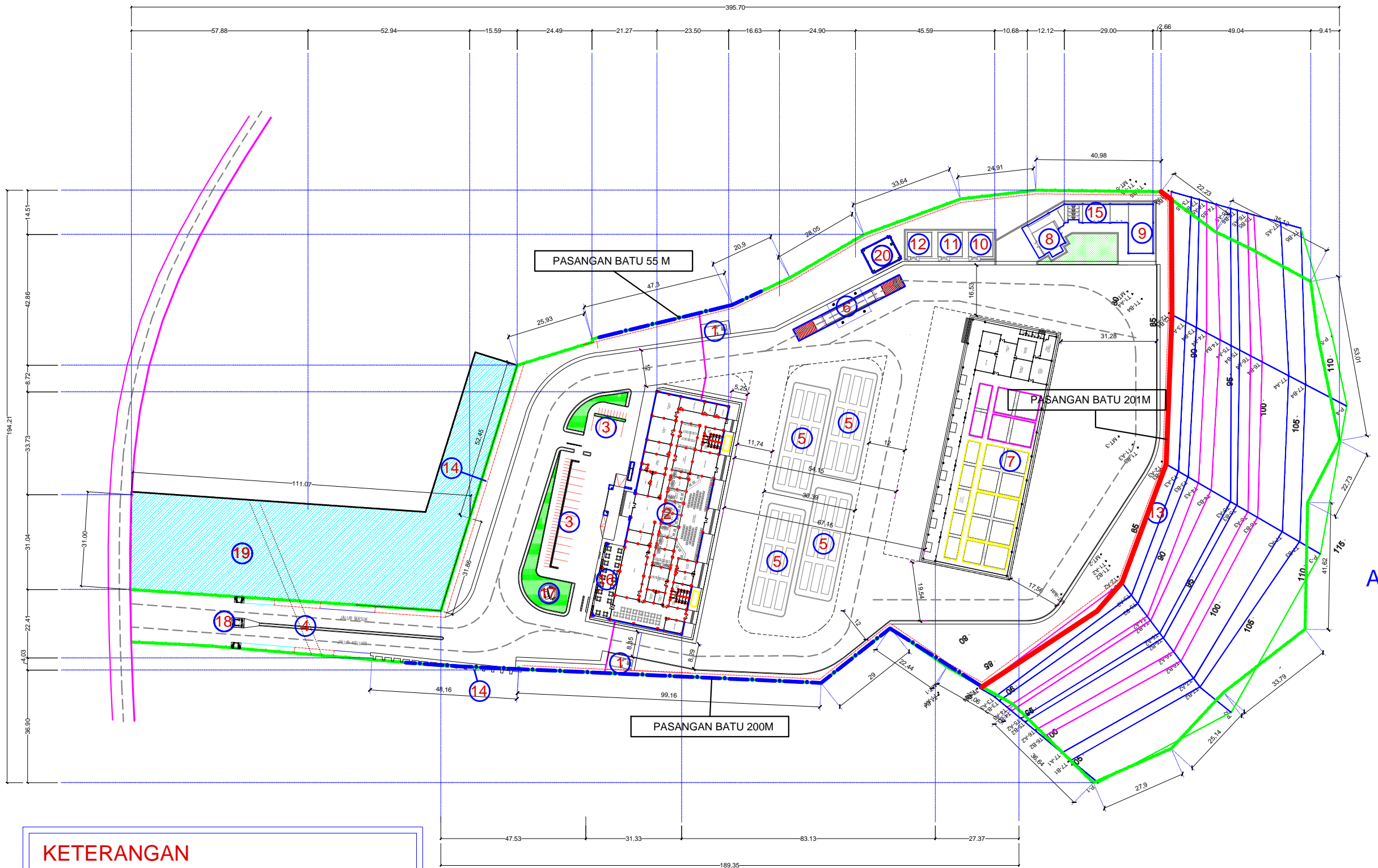
LAYOUT RENCANA PASANGAN BATU SKALA 1 : 1400
