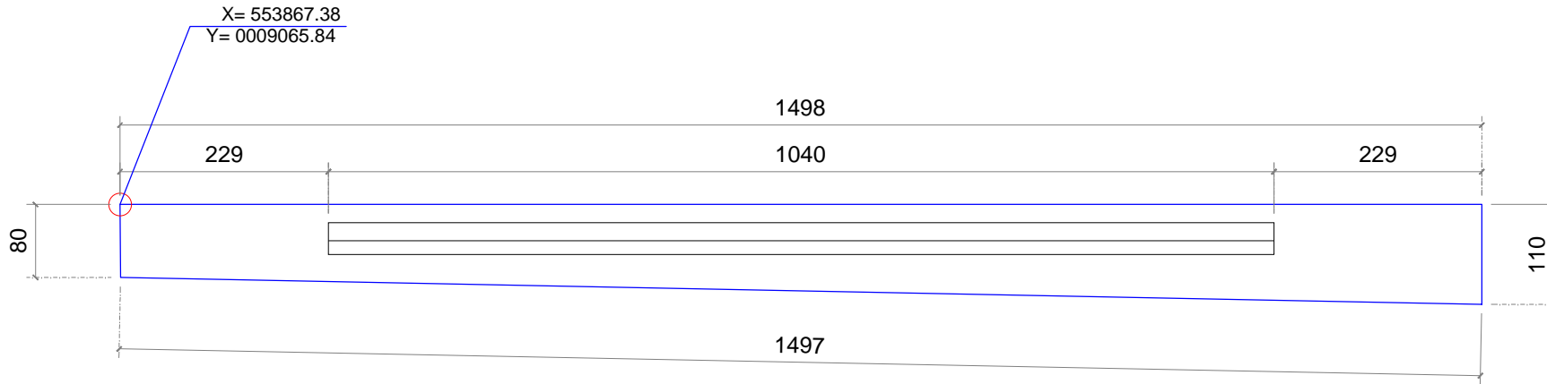
DENAH PLANK NAMA SKALA 1:50
