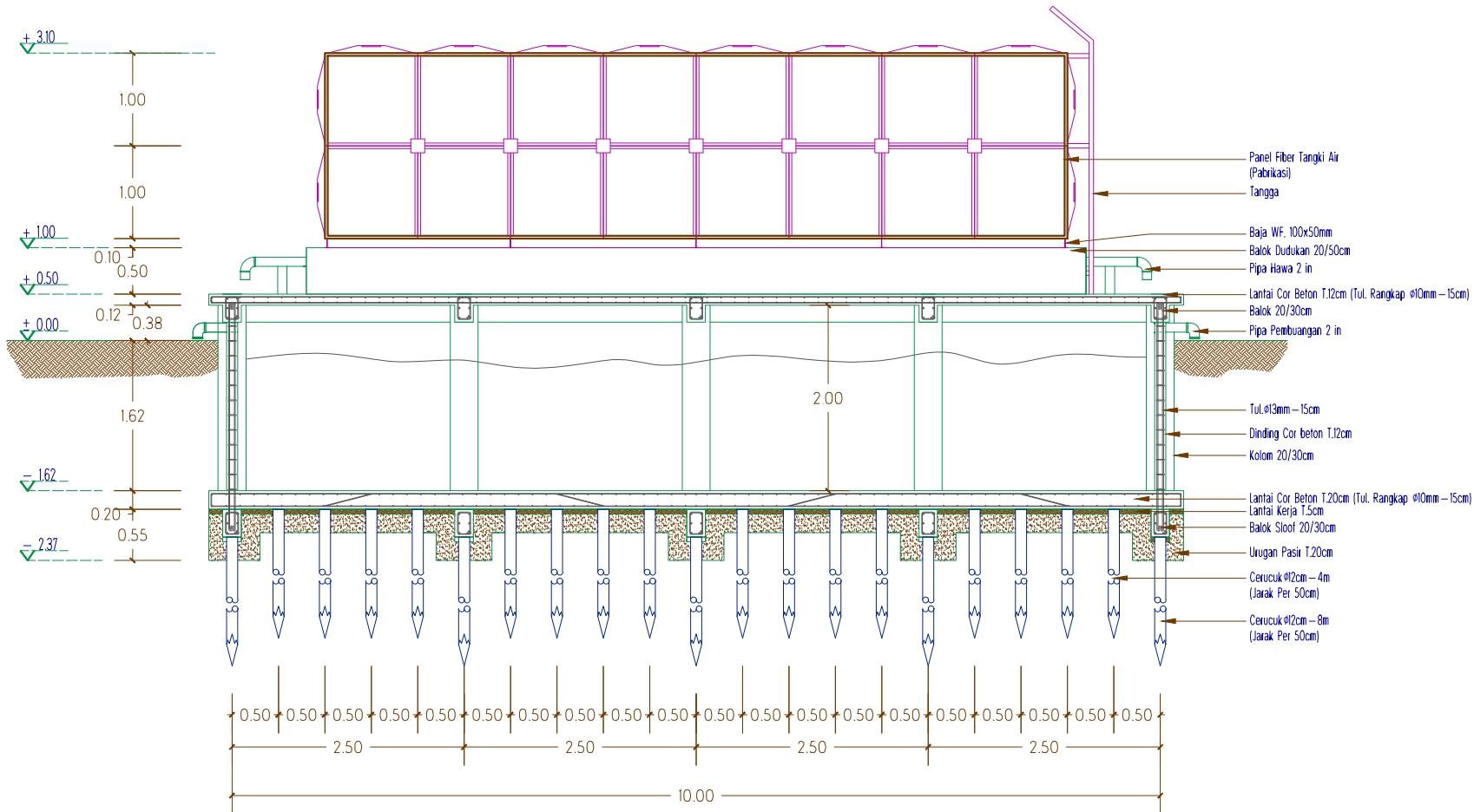
POTONGAN - A SKALA 1:50
