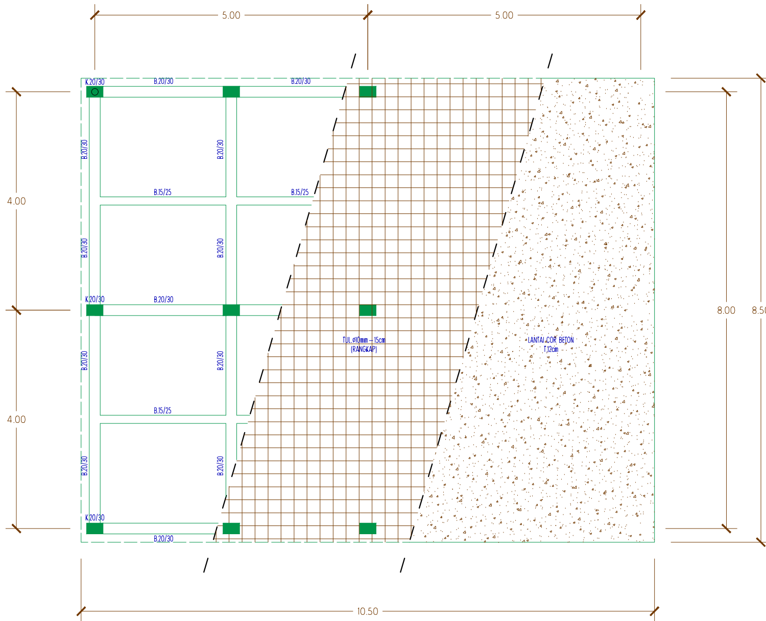
RENCANA LANTAI ATAS SKALA 1:50
