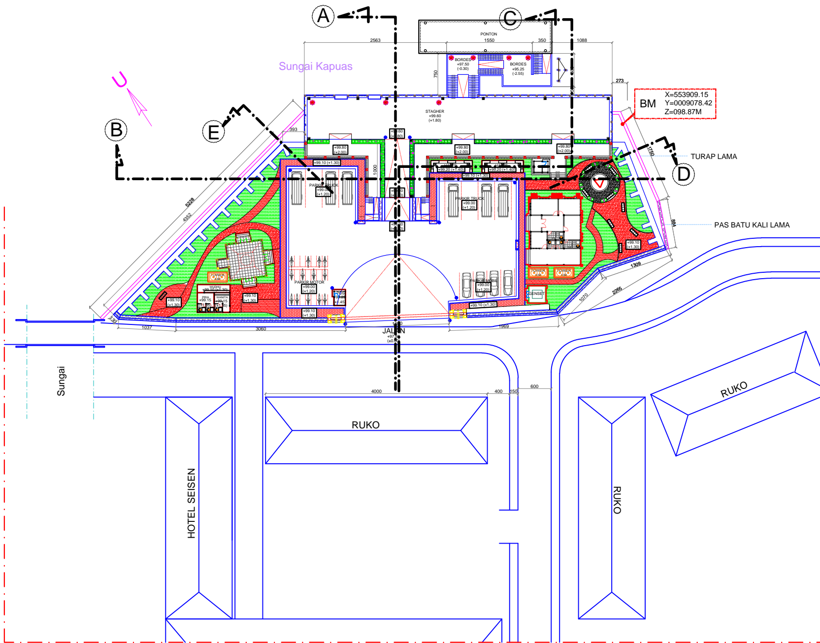
LAYOUT PLAN RENCANA DERMAGA SUNGAI DURIAN
