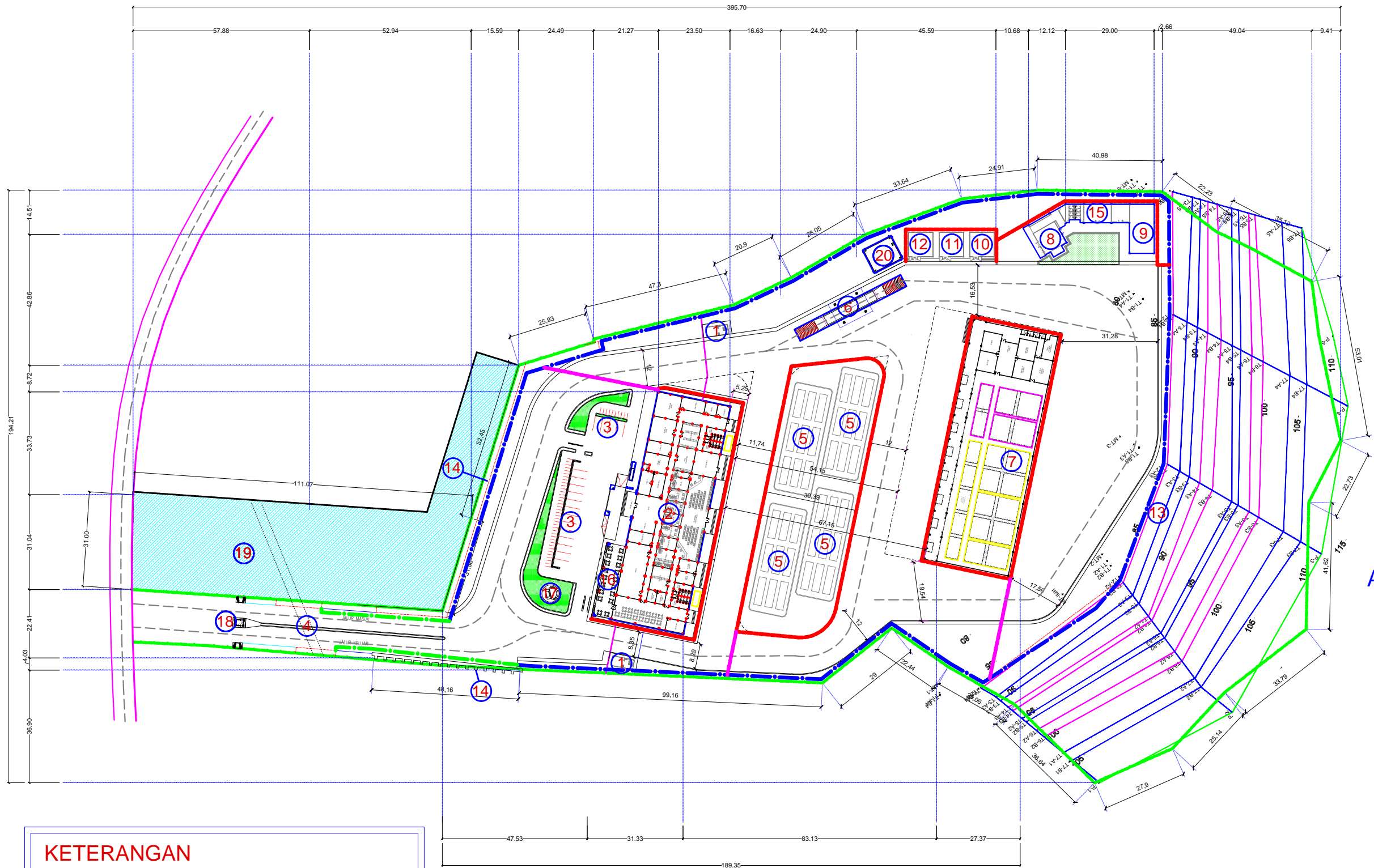
LAYOUT RENCANA SALURAN KAWASAN SKALA 1 : 1400
