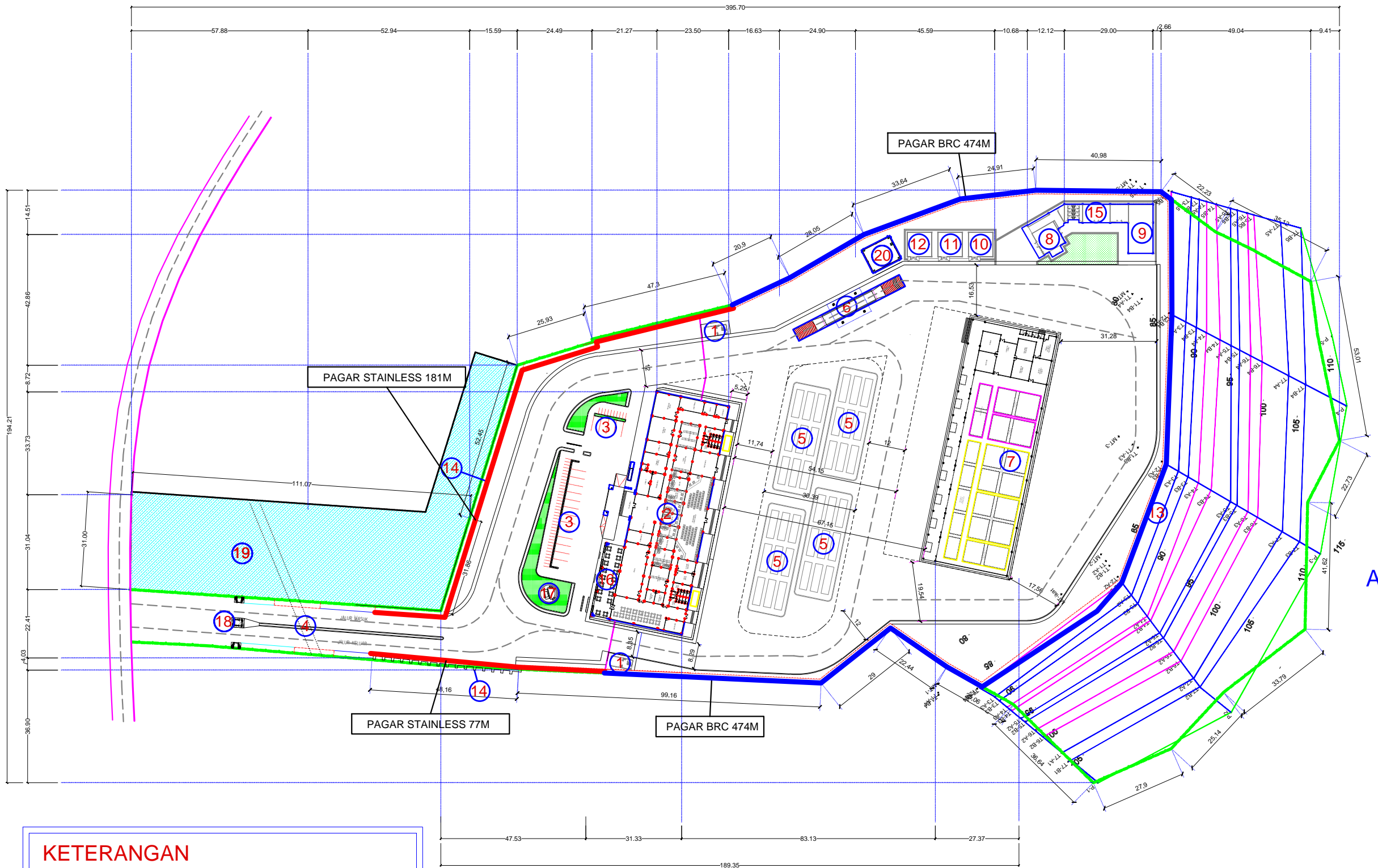
LAYOUT RENCANA PEMASANGAN PAGAR SKALA 1 : 1400
